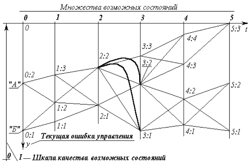
Рис. 7. Динамическое программирование, Различение и достаточно общая теория управления
