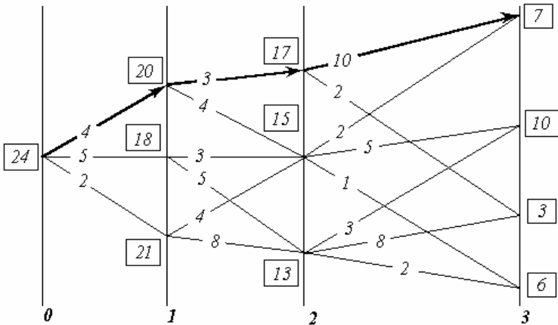
Рис. 6. К СУЩЕСТВУ МЕТОДА ДИНАМИЧЕСКОГО ПРОГРАММИРОВАНИЯ. ОПТИМАЛЬНАЯ ТРАЕКТОРИЯ.
