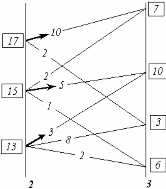
Рис. 5. К существу метода динамического программирования. Анализ переходов.
